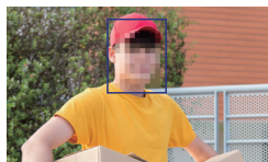
人脸
