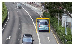
逆行
